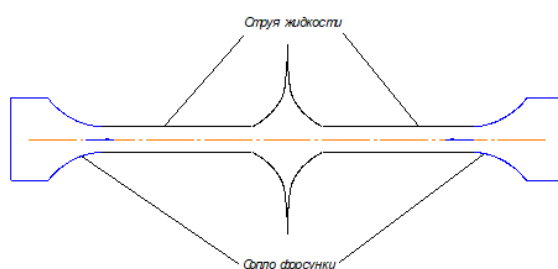
Рис.4. Форсунки с соосным расположением
