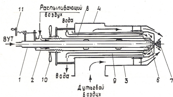
Рис.3. Форсунка для ВУТ: 1 – трубка для ВУТ, 2 – трубка для распыливающего воздуха, 3 – корпус, 4 – канал подвода дутьевого воздуха, 5 – винтовой завихритель, 6 – рассекатель, 7 – канал подвода охлаждающей воды, 8 – канал отвода охлаждающей воды, 9 – механизм перемещения винтового завихрителя, 10 – ограничительный винт
