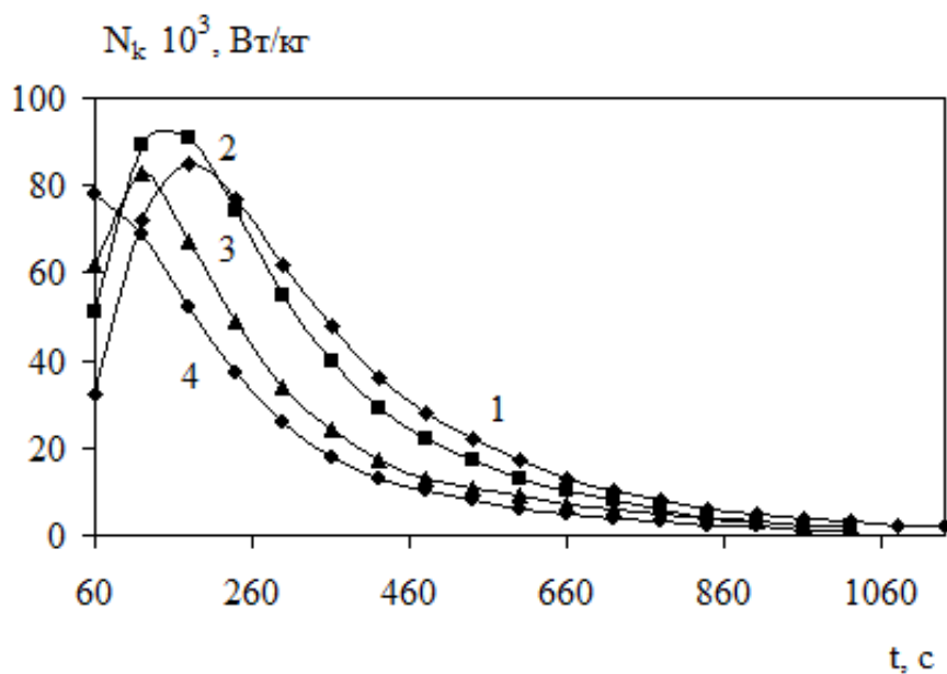
Рис.3. Зависимость удельной мощности тепловыделения при изотермической кристаллизации из закалённого состояния пентапласта от времени ( 1 - T_{кр} = 314 \text{ K} ; 2 - T_{кр} = 319 \text{ K} ; 3 - T_{кр} = 325 \text{ K} ; 4 - T_{кр} = 331 \text{ K} )
