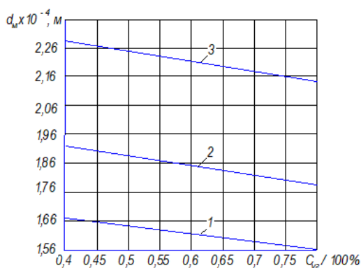
Рис. 2. Зависимость медианного диаметра капель от концентрации угля в ВУТ при различных значениях динамической вязкости топлива: 1 – \eta_{жс} = 1,0 Па·с; 2 – \eta_{жс} = 1,4 Па·с; 3 – \eta_{жс} = 2,5 Па·с.
