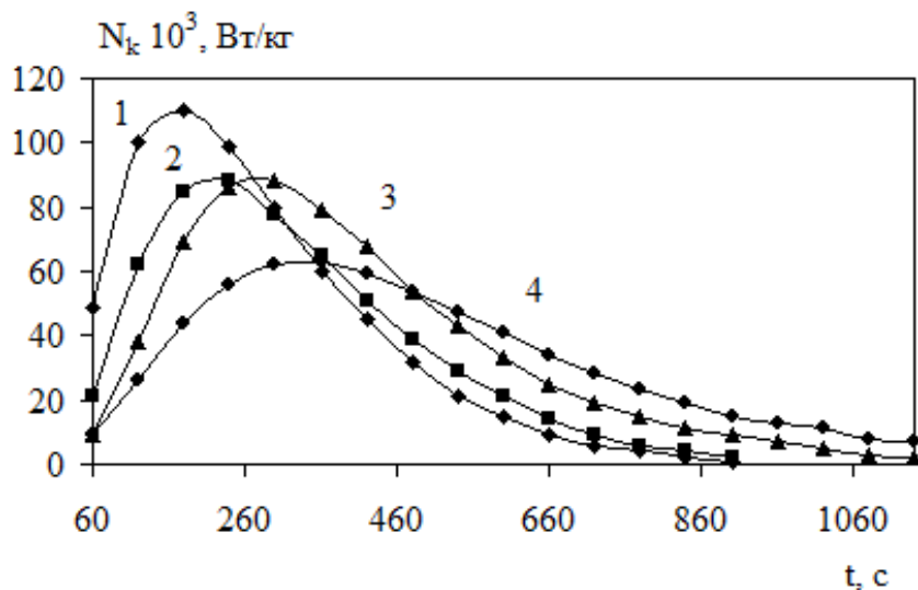
Рис.2. Зависимость удельной мощности тепловыделения при изотермической кристаллизации из расплава пентапласта от времени ( 1 - T_{кр} = 394,5 \text{ K} ; 2 - T_{кр} = 400 \text{ K} ; 3 - T_{кр} = 402,5 \text{ K} ; 4 - T_{кр} = 406,5 \text{ K} )
