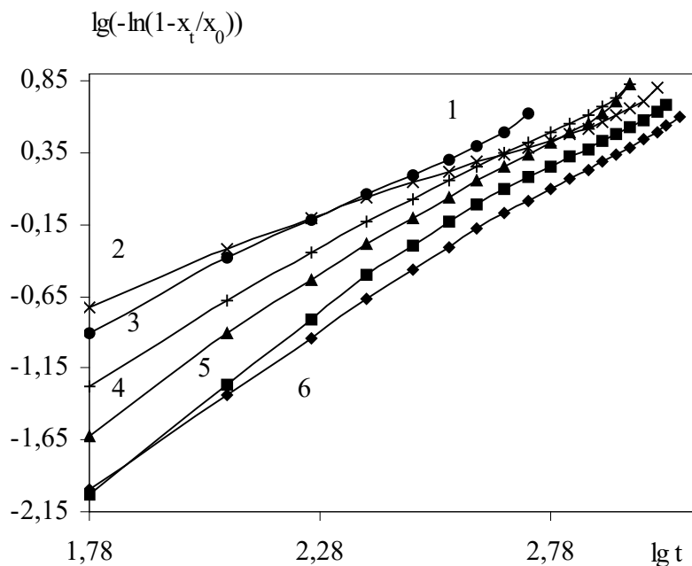
Рис. 1. Изотермы кристаллизации пентапласта из закалённого состояния при T_{кр} = 331\text{ K} (1) и T_{кр} = 325\text{ K} (2) и из расплава при T_{кр} = 394,5\text{ K} (3), T_{кр} = 400\text{ K} (4), T_{кр} = 402,5\text{ K} (5) и T_{кр} = 406,5\text{ K} (6)
