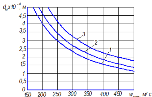
Рис.1. Зависимость медианного диаметра капель от относительной скорости \omega_{отн} при различных значениях динамической вязкости топлива: 1 – \eta_{жс} = 1,0 Па·с; 2 – \eta_{жс} = 1,4 Па·с; 3 – \eta_{жс} = 2,5 Па·с.
