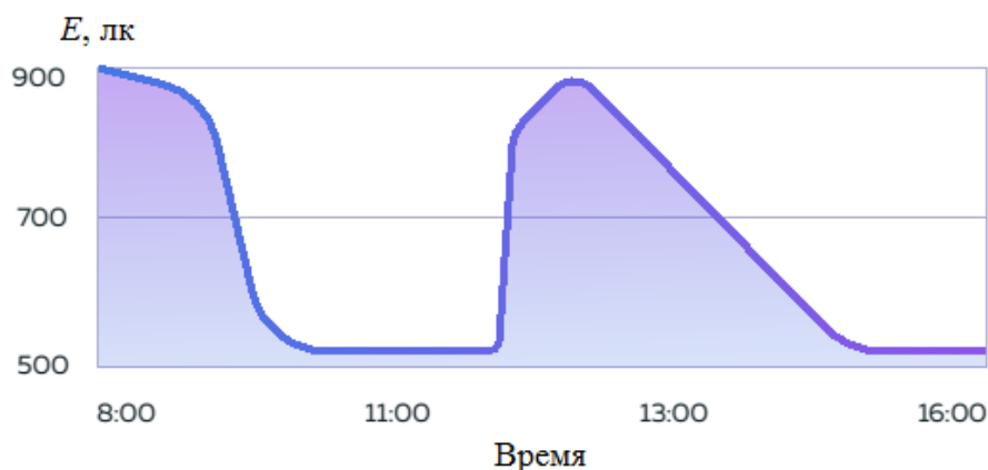
Рис. 5. Пример реализации биодинамического освещения
