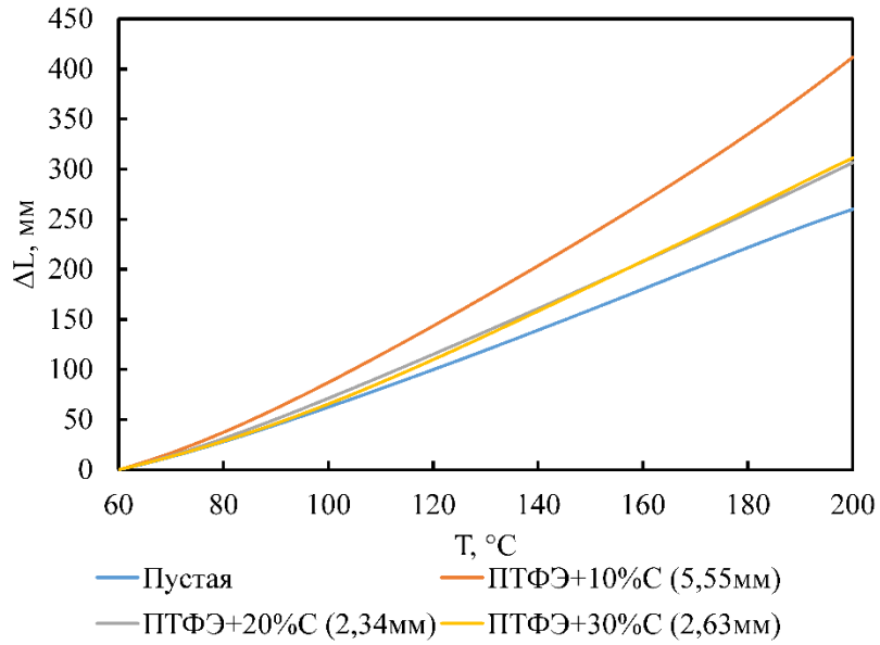
Рис. 1. Зависимости относительного удлинения образцов от температуры
