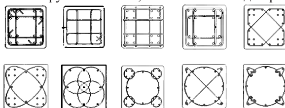
Рис. 1. Новые виды косвенного армирования колонн
