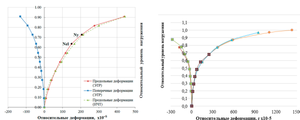
Рис. 4. Диаграммы деформирования трубобетонных элементов: а – класс B-40; б – класс SA-80
