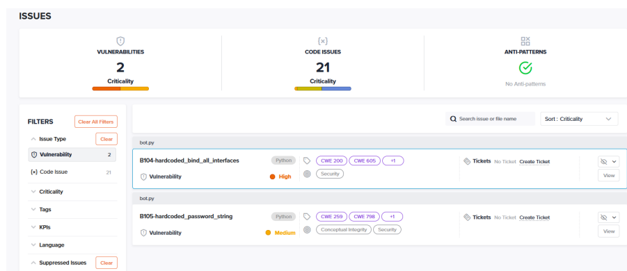
Рис. 2. Пример анализа кода с GitHub инструментами Embold
