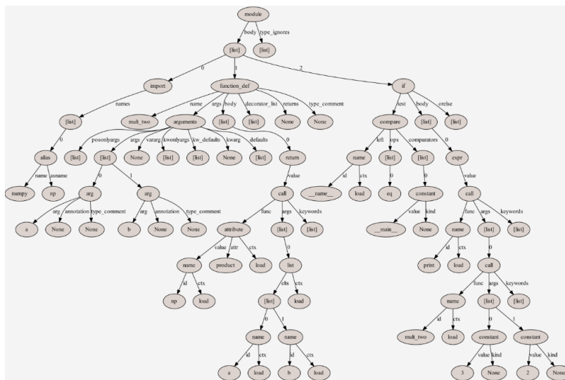
Рис. 1. Пример абстрактного синтаксического дерева
