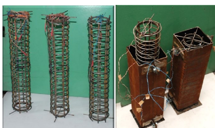
Рис. 3. Опытные образцы трубобетонных элементов
