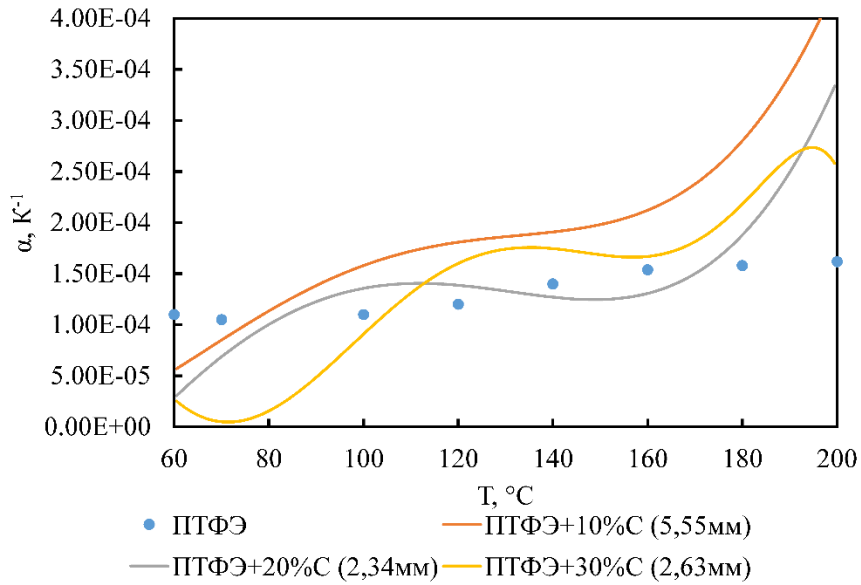
Рис. 2. Зависимости ТКЛР образцов от усредненной температуры
