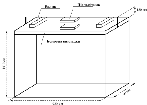
Рис. 5. Конструкция армстола
