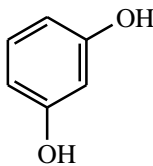
резорцин
