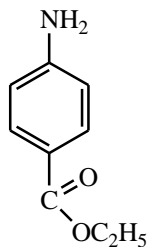
анестезин
