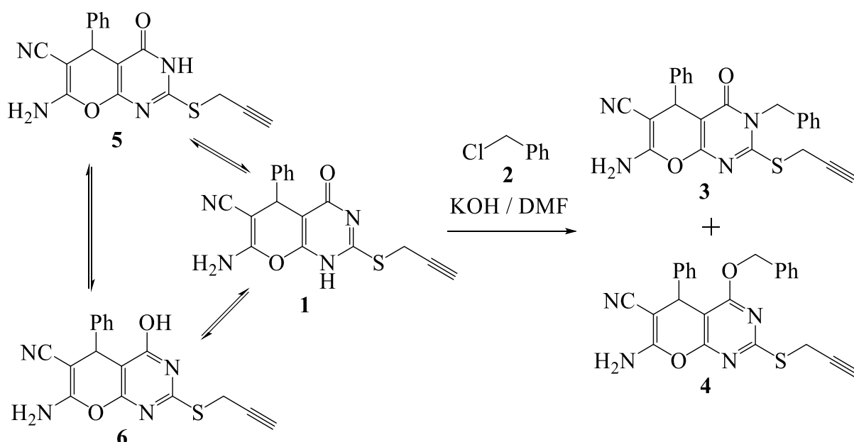
Схема 1. Бензилирование замещенного пирано[2,3- d ]пиримидина 1 .
