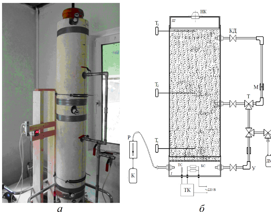
Рис. 2. Установка для исследования переноса радона в пористых средах: а) внешний вид; б) схема: НК – камера накопительная; П – ротаметр; T_1 - T_3 – термометры погружные; ТК – термоконтроллер; ТС – термосопротивление; БС – блок сопротивлений; КД – кран двухходовой; Т – кран трехходовой; У – переходник угловой 90°; К – компрессор; М – муфта; ДМ – манометр дифференциальный
