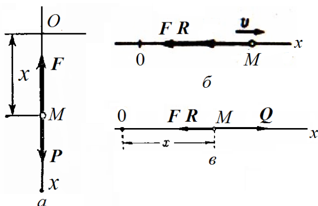
Рис. 1. Схемы механических колебательных процессов: а) свободные колебания; б) свободные затухающие колебания; в) вынужденные затухающие колебания
