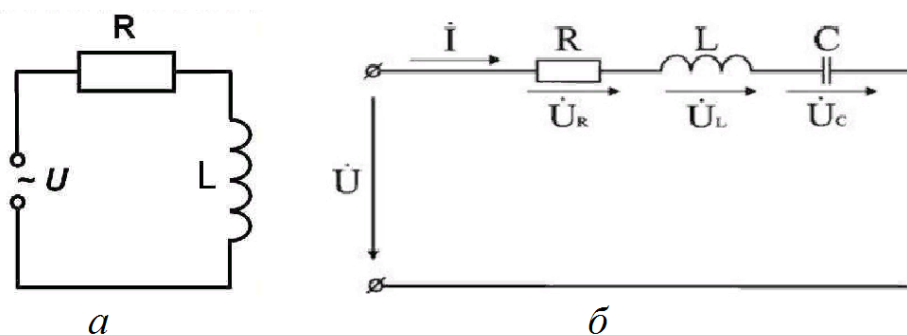
Рис. 2. Цепи переменного тока: а) с активным и индуктивным сопротивлением; б) колебательный контур
