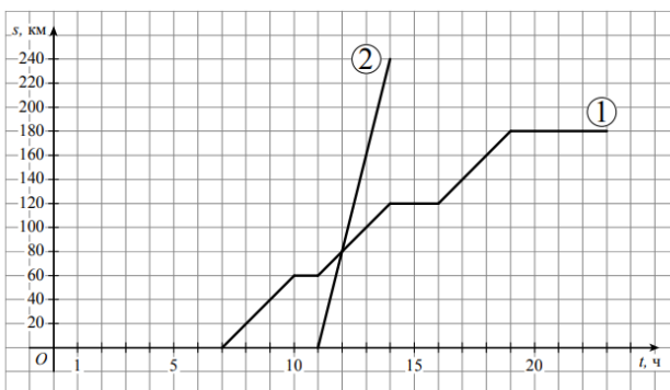
Рисунок 1 – График движения велосипедиста и автомобиля
