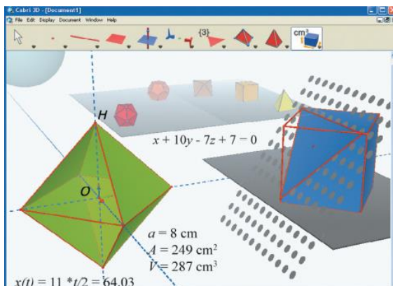
Рисунок 2 – Интерфейс программыCabriExpress
